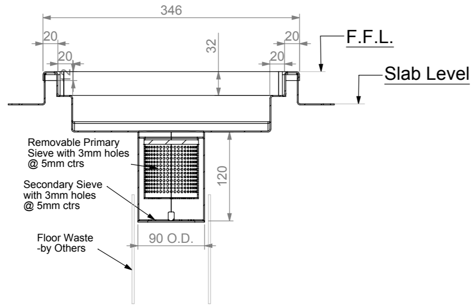
SECTION T-T SCALE 1 : 5
